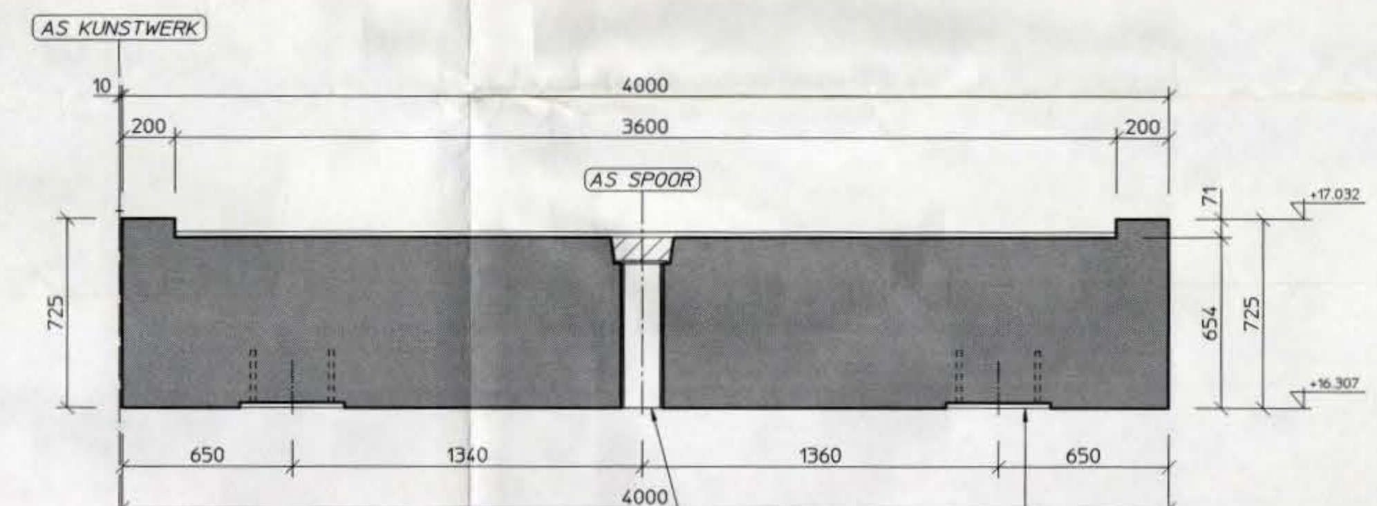
Doorsnede C-C Schaal 1:20
