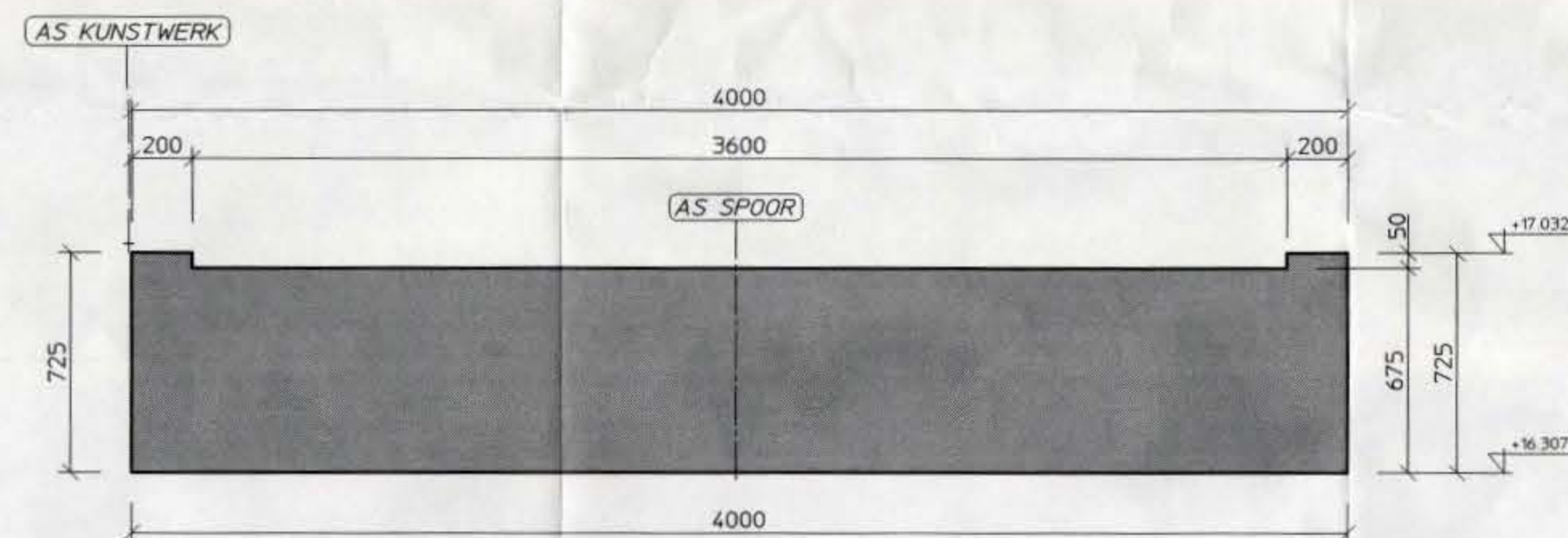
Doorsnede B-B Schaal 1:20
