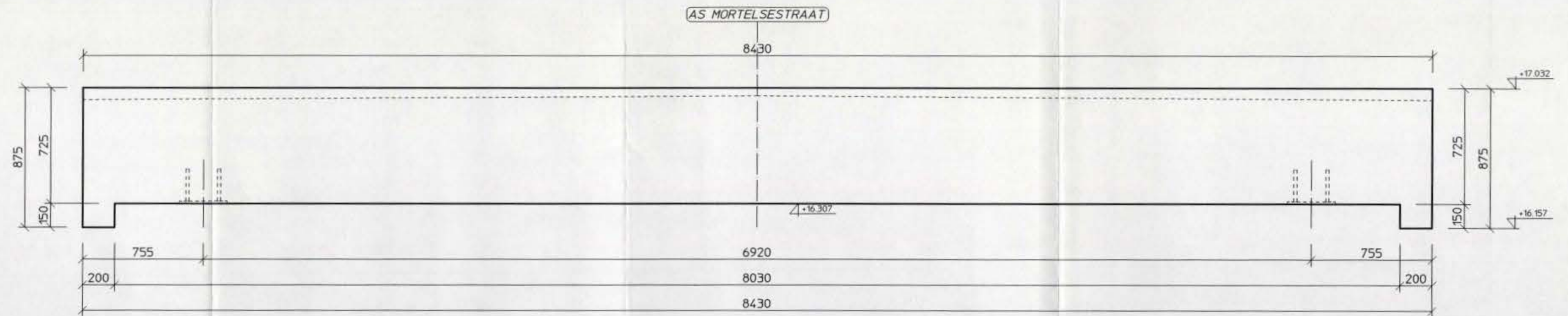
Vooraanzicht Schaal 1:20
