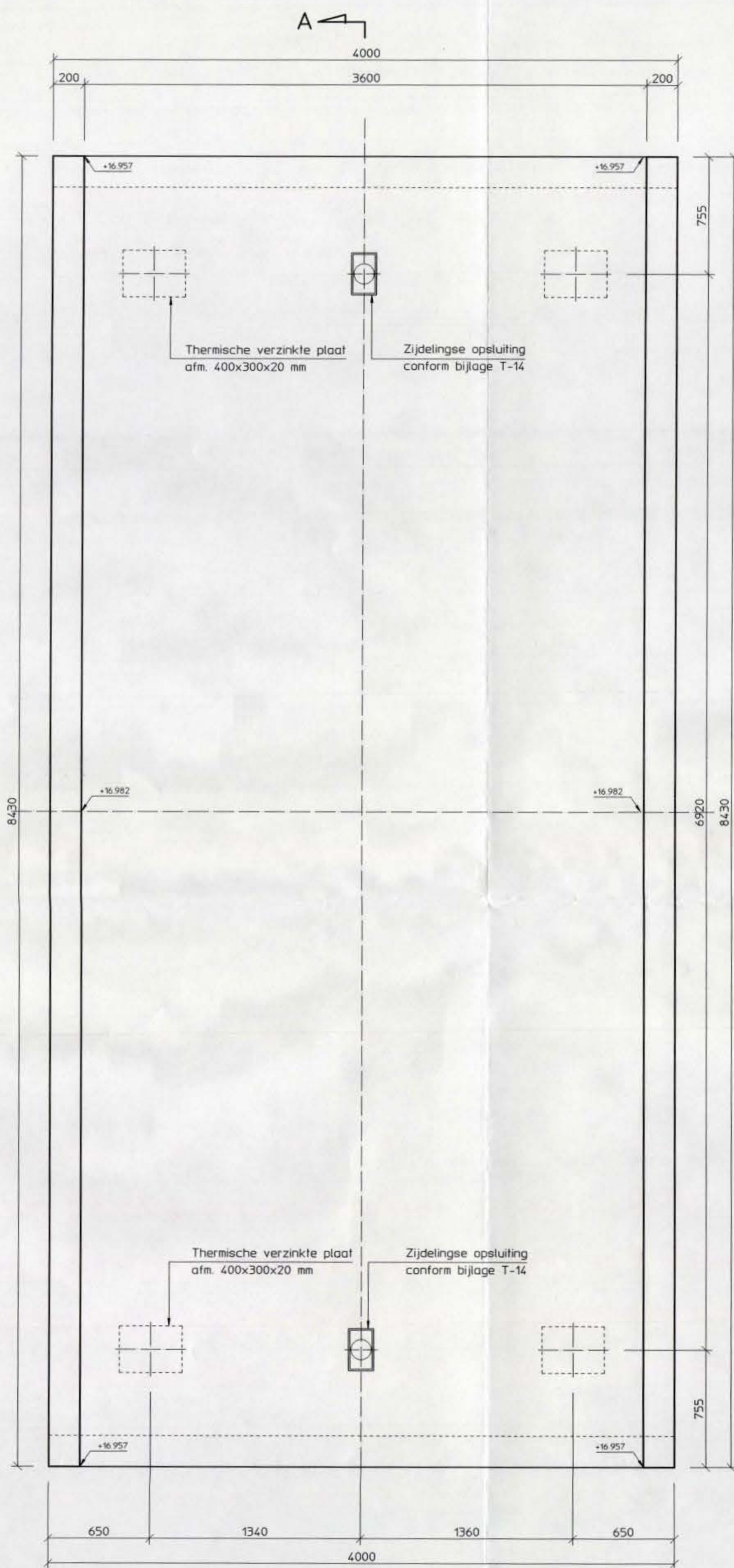
Bovenaanzicht Schaal 1:20
